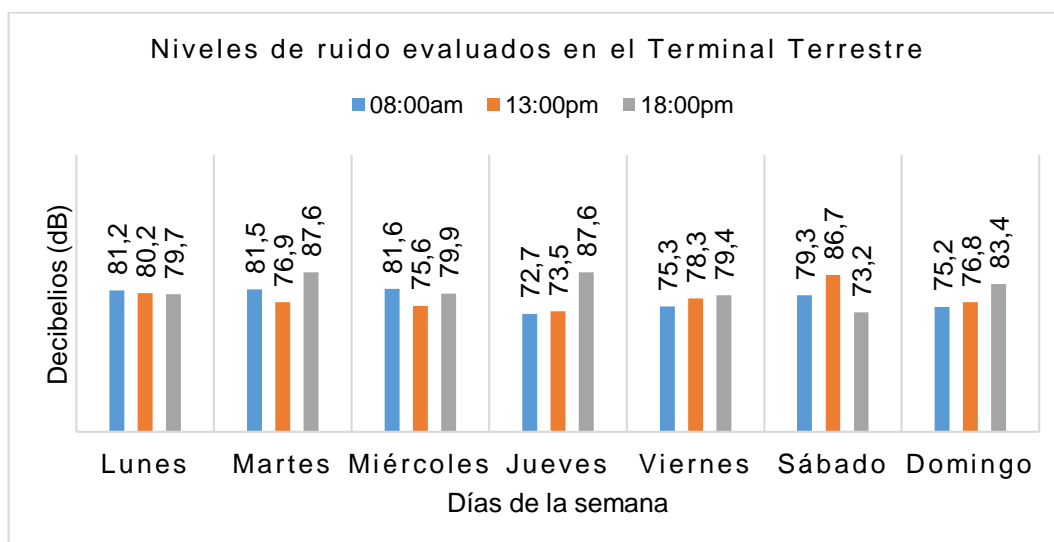
Figura 3. Evaluación de ruido ambiente en el Terminal Terrestre, Av. Abraham Calazacón.
