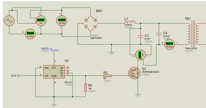
Figura 8. Circuito de potencia
