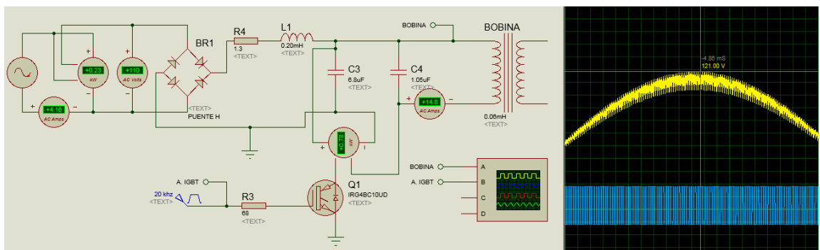
Figura 5. Simulación del circuito 20KHz, capacitor 1.05uF
