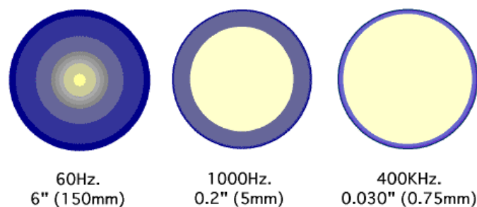
Figura 2. Efecto piel en una pieza cilíndrica de acero (MohammadHosseinTavakoli, 2011)
