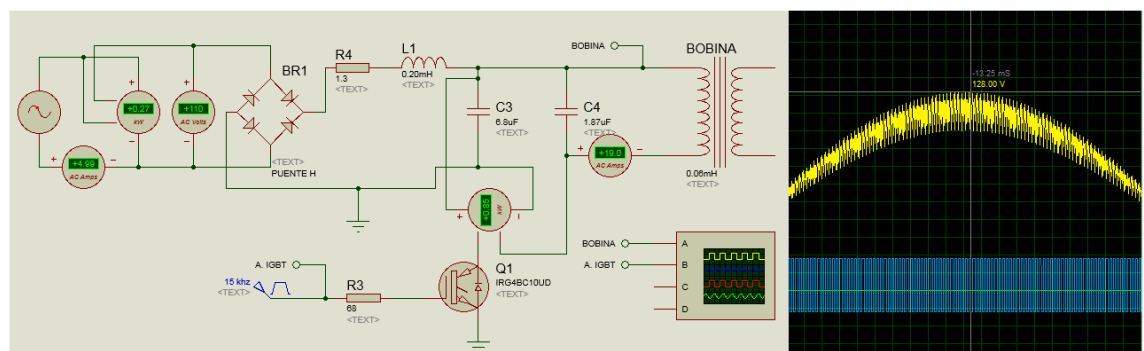
Figura 6. Simulación del circuito 15KHz, capacitor 1.87uF
