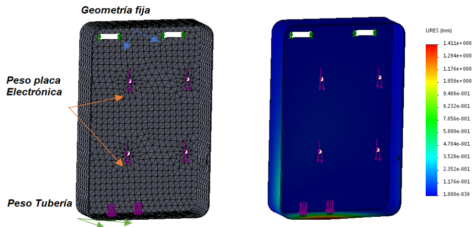
Figura 10. Análisis de elementos finitos de la carcasa
